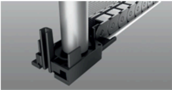
Parte inferior de caja - guía de retención
