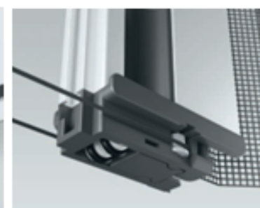
Dos poleas laterales a laderecha e izquierda.
