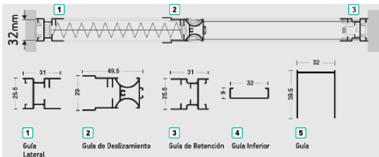
UNA SOLA HOJA LATERAL ancho máx: 2.000mm altura máx: 3.000mm
