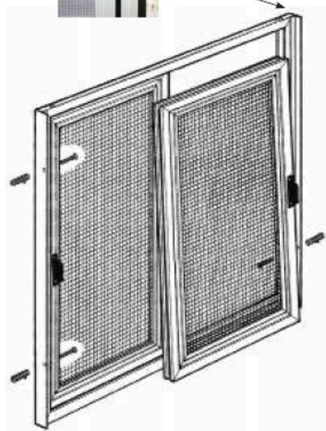
Detalle mosquitera
